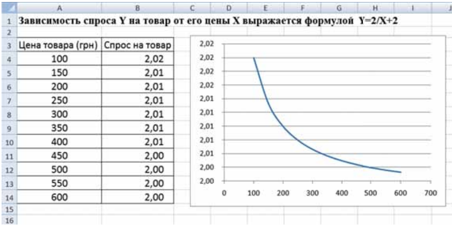
Рис. 7.9. Точечная диаграмма
