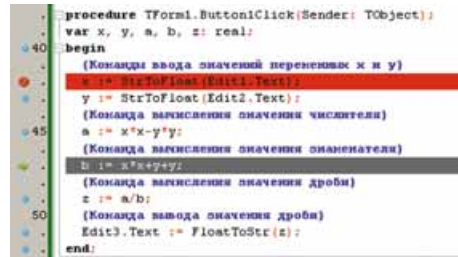
Рис. 6.13. Пошаговое исполнение
