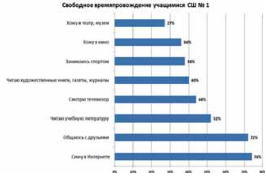
Рис. 7.7. Линейчатые диаграммы
