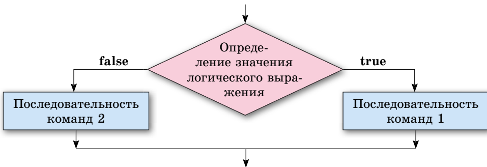
Рис. 6.22. Полное ветвление
