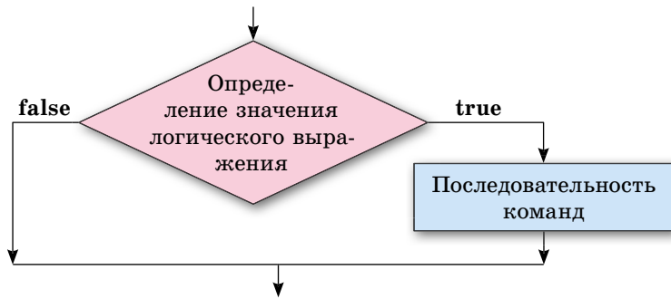
Рис. 6.23. Неполное ветвление
