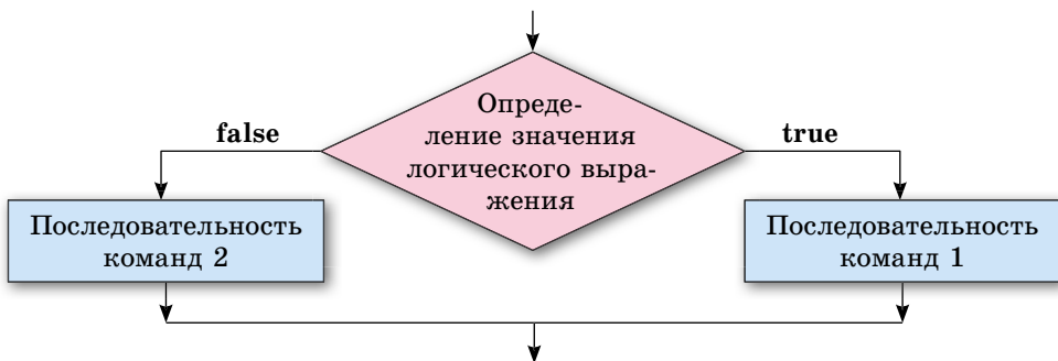
Рис. 6.18. Полное ветвление
