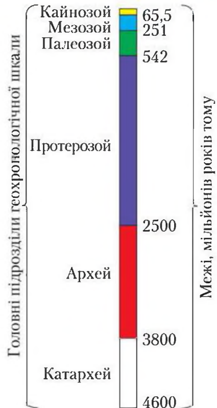
Рис. 62.2. Геохронологічна шкала
