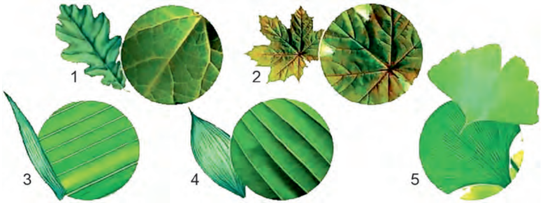
Жилкування листків: пірчасте (1), пальчасте (2), паралельне (3), дугове (4), вилчасте (5)
