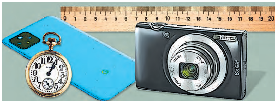
Засоби та прилади, що можуть стати в пригоді під час проведення дослідження
