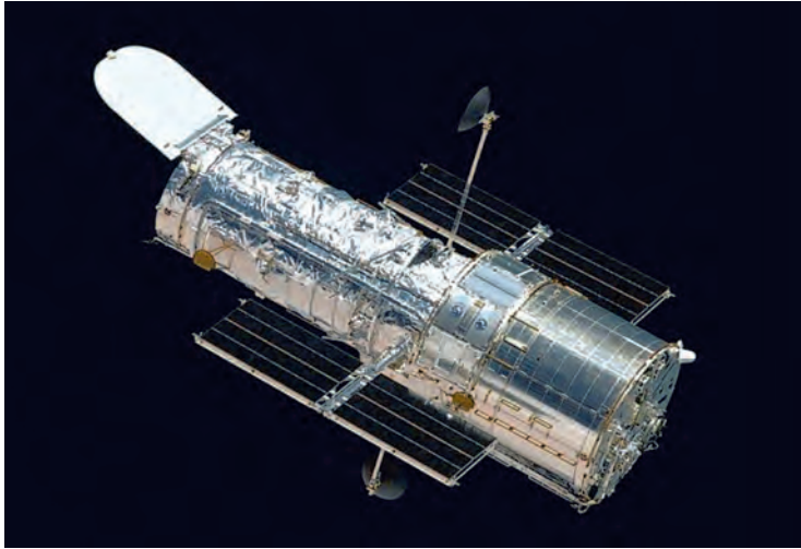
Телескоп «Габбл» на орбіті Землі. Світлина зроблено з космічного корабля «Атлантис» у 2009 році
