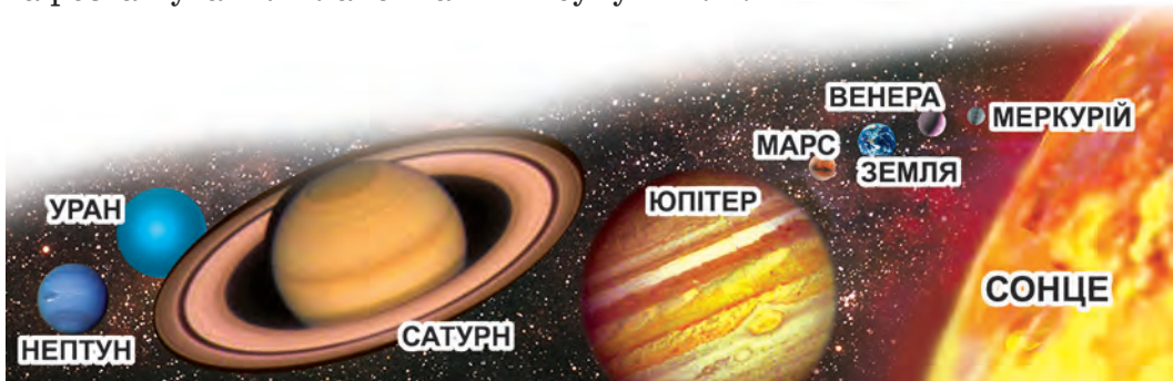
Планети у складі Сонячної системи. Відносні розміри планет збережені, але їх зображення зіставлені поруч
