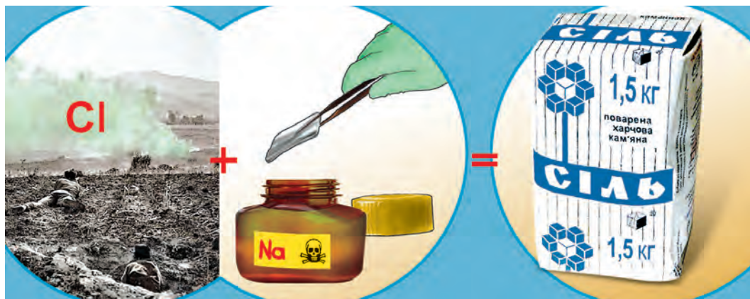
Звичайна кухонна сіль утворена атомами Хлору й Натрію
