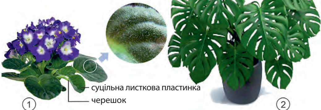
Кімнатні рослини, що походять із тропіків: сенполія (1) та монстера (2)
