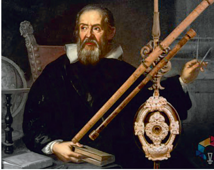
Галілео Галілей (1564–1642) зі створеним ним телескопом
