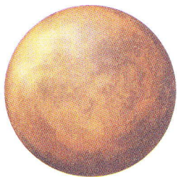
Венера
