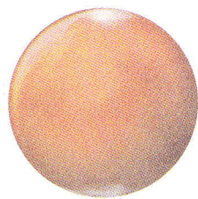
Марс
