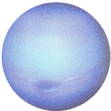
Нептун
