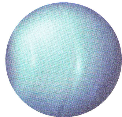
Уран
