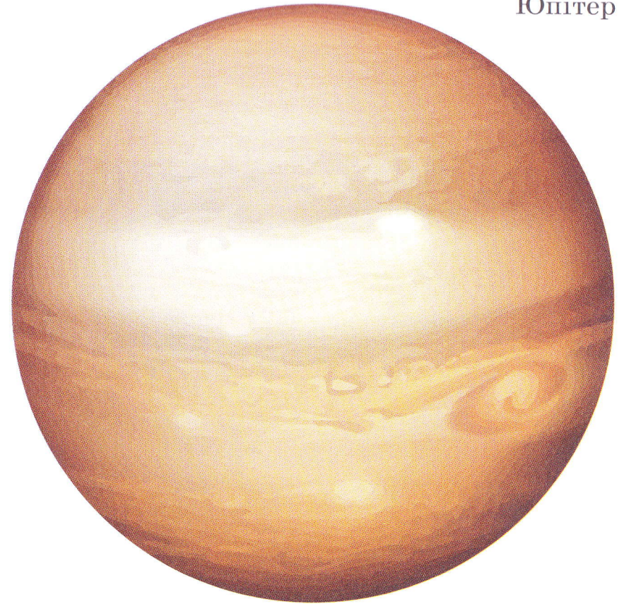
Юпітер
