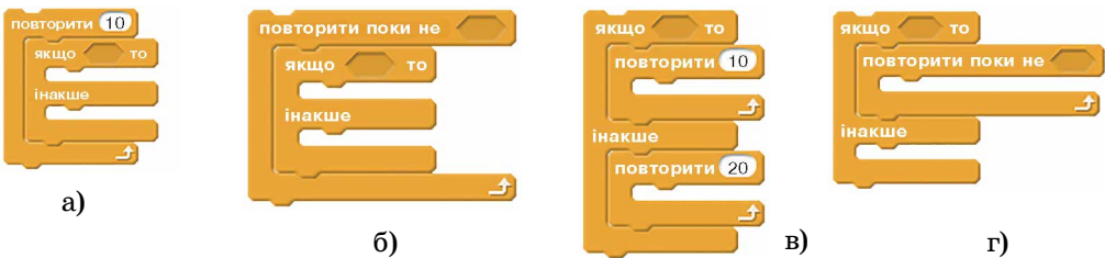
Мал. 3.46. Вкладені цикли і розгалуження в Scratch 2
