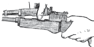
9. Відокремити газову трубку зі ствольною накладкою
