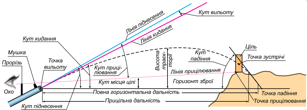
Елементи траєкторії
