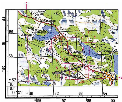
Визначення прямокутних координат точки за картою (точка В)
