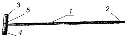
Приладдя автомата, підготовлене для чистки: 1 – шомпол; 2 – протирка; 3 – пенал; 4 – викрутка; 5 – головка шомпола
