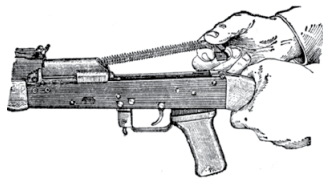
6. Відокремити зворотний механізм
