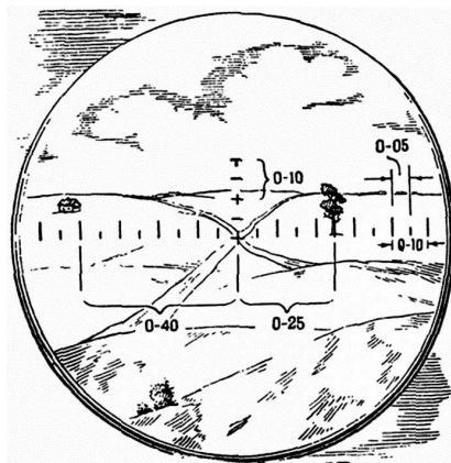
Сітка бінокля: маленька поділка дорівнює 5 тисячним, велика – 10 тисячним
