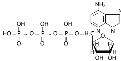
Структурная формула АТФ (химическая формула – C_{10}H_{16}N_5O_{13}P_3 )
