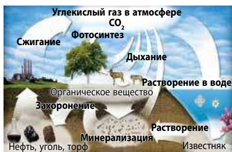
Ил. 165. Круговорот CO_2 в биосфере
