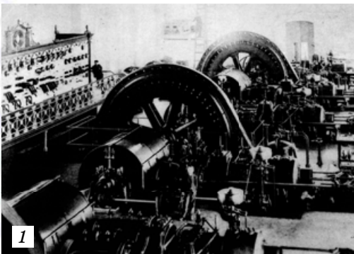
1 – Друга електрична станція на Дніпровському заводі в с. Кам'янське Катеринославської губернії. Початок початку XX ст.
